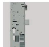
ES 1772 5-FACH VERRIEGE- LUNG, M-TS* KOMPATIBEL MIT ZUTRITTSSYSTEM: 1
